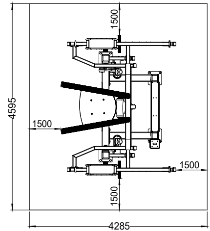
Güvenlik ve Kullanım Alanı Safety and Usage Area
