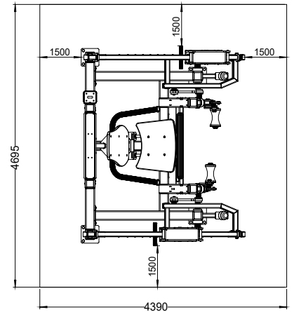
Güvenlik ve Kullanım Alanı Safety and Usage Area
