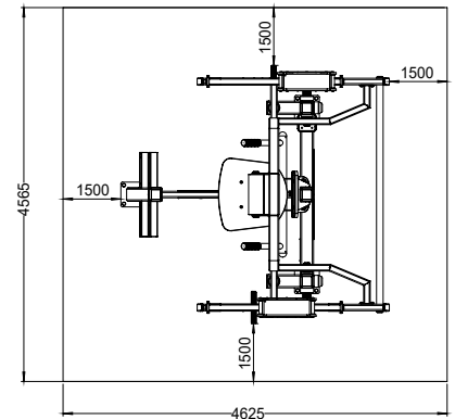
Güvenlik ve Kullanım Alanı Safety and Usage Area
