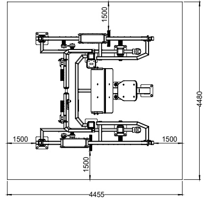
Güvenlik ve Kullanım Alanı Safety and Usage Area
