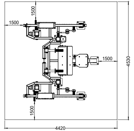
Güvenlik ve Kullanım Alanı Safety and Usage Area
