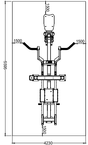
Güvenlik ve Kullanım Alanı Safety and Usage Area
