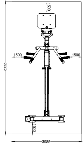
Güvenlik ve Kullanım Alanı Safety and Usage Area
