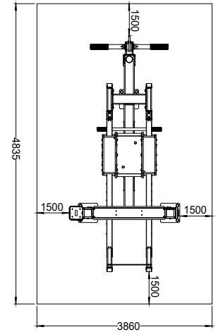
Güvenlik ve Kullanım Alanı Safety and Usage Area
