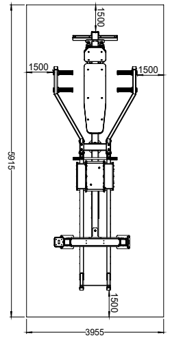
Güvenlik ve Kullanım Alanı Safety and Usage Area
