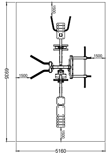
Güvenlik ve Kullanım Alanı Safety and Usage Area
